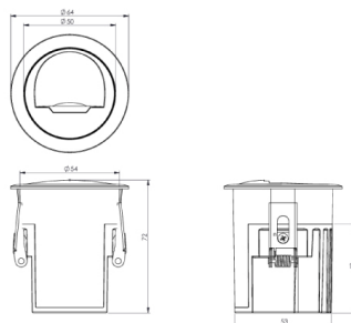
Vion Wall Washer 60
